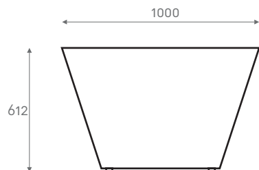
Kónica100 Código: JAR-134/C Volumen: 300 lt. Peso: 65 kg.
