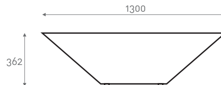
Kónica130 Código: JAR-134/D Volumen: 200 lt. Peso: 70 kg.
